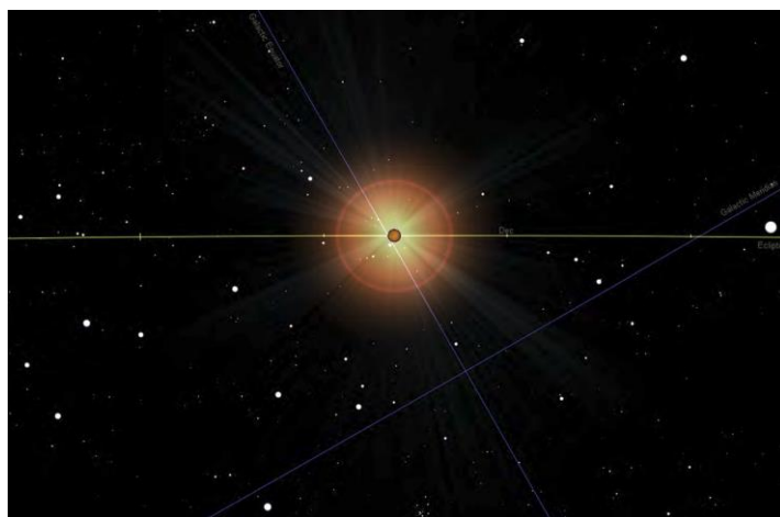
Fig. 14: La posizione del Sole il 21 dicembre 2012: pur trovandosi quasi sull'equatore galattico (la linea blu quasi verticale), esso si proietta a notevole distanza dal meridiano galattico (la linea blu perpendicolare alla prima), e quindi dal centro della nostra Galassia. La linea gialla è l'eclittica (immagine realizzata col software Starry Night pro plus 6)
