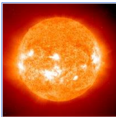
Fig. 1: Immagine della superficie del Sole presa da SOHO, la nave spaziale ESA-NASA: la navicella, lanciata nel dicembre 1995, controlla costantemente il Sole.
